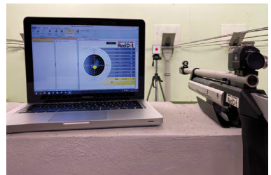
Lichtgewehr mit Auswertung am Laptop
